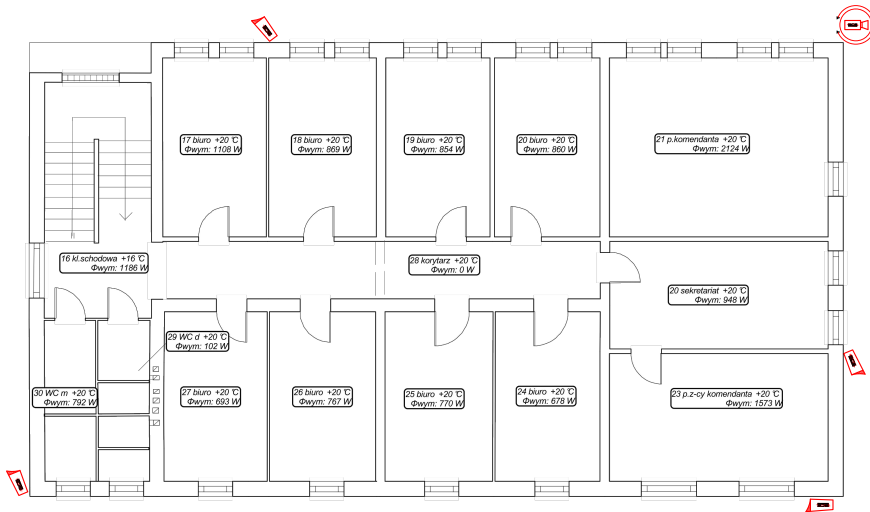
RZUT PIĘTRA I SKALA 1 : 100
