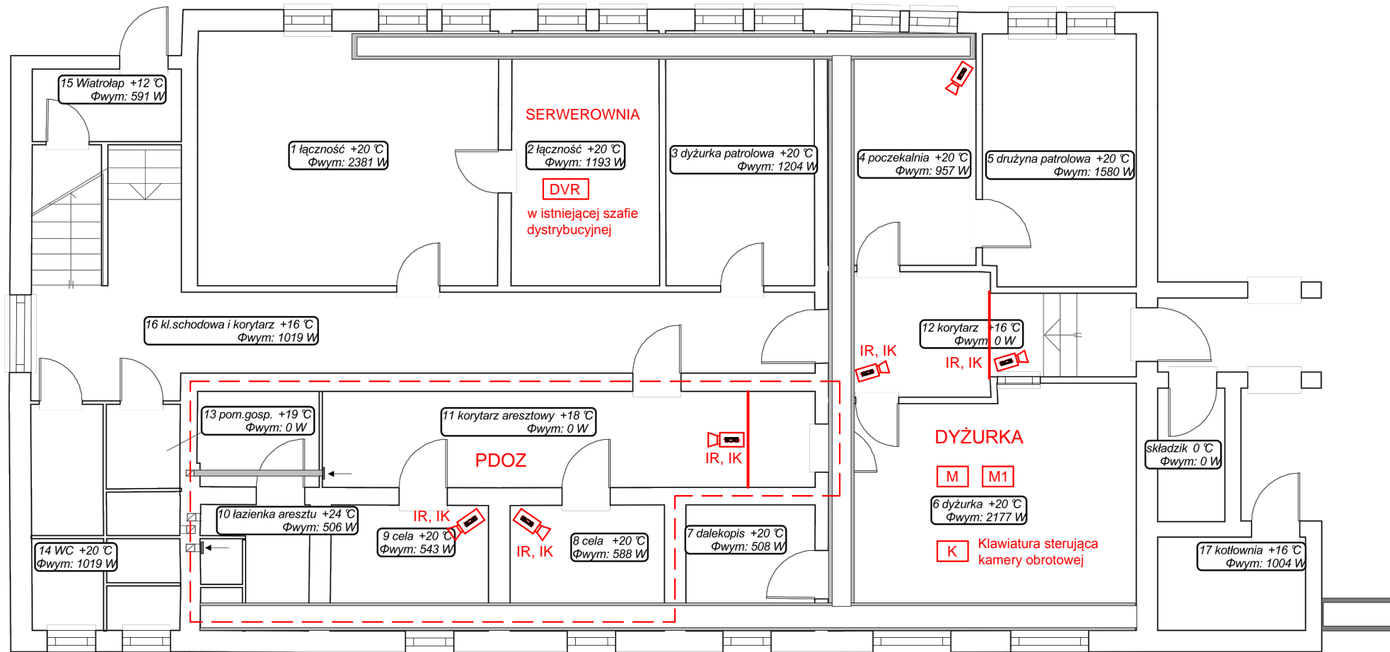
RZUT PARTERU SKALA 1 : 100
