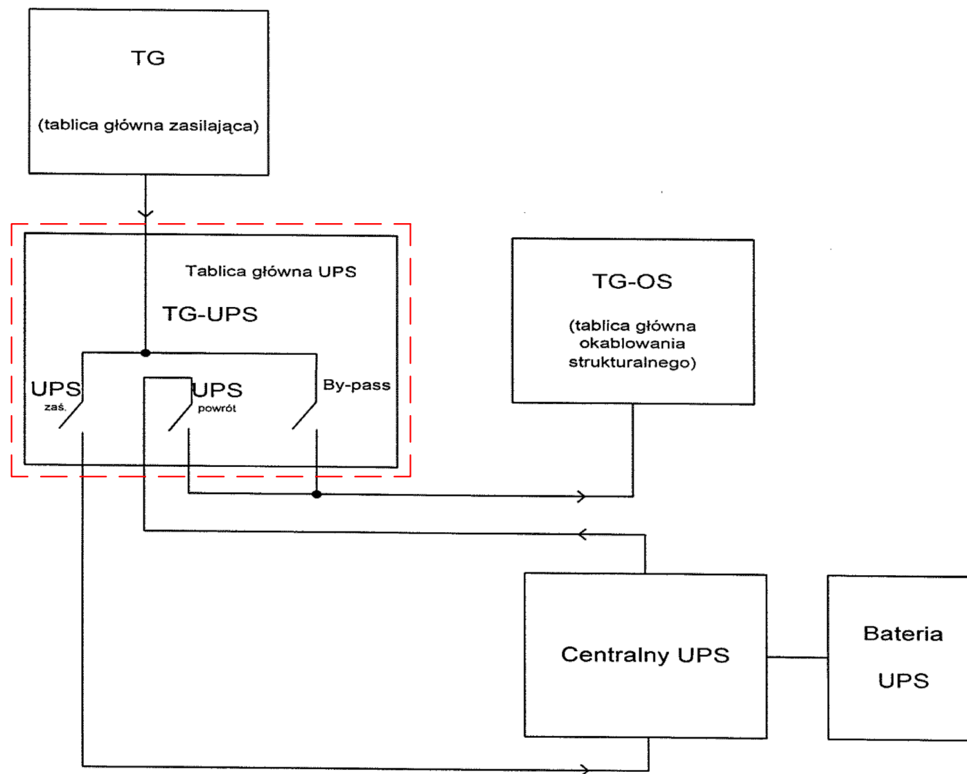
Rysunek przedstawiający koncepcję BY-PASS-u.
